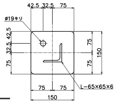
9tベースプレート詳細圖
