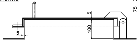
マンホール詳細圖
