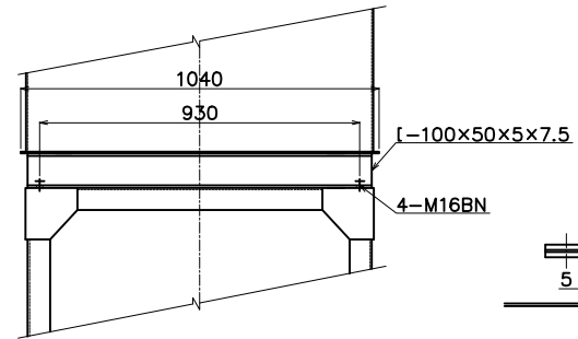
A - A 矢視圖
