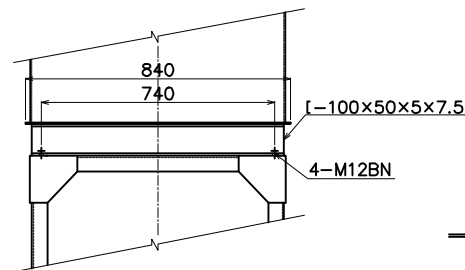
A - A 矢視図
