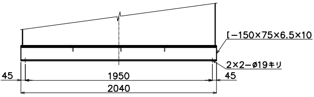
A-A矢視図
